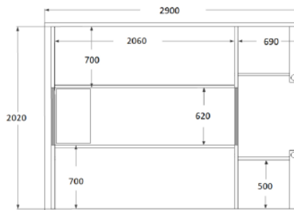
Plantegning
